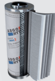
Darstellung mehrlagiger Aufbau EXAPOR®MAX 3
