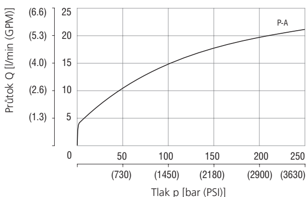
Výkonová charakteristika SD2P-B4/H3Y13-5
