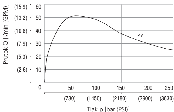
Výkonová charakteristika SD2P-B4/H3Y13-25
