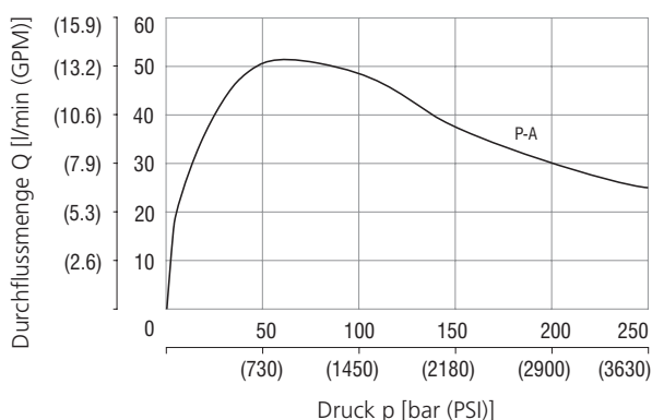
Leistungskennlinie SD2P-B4/H3Y13-25
