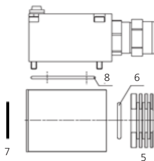
Dichtungssatz für den elektrischen Teil des Ventils
