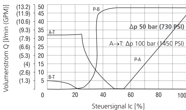
Leistungskennlinie SD2P-B4/H3Y13-25
