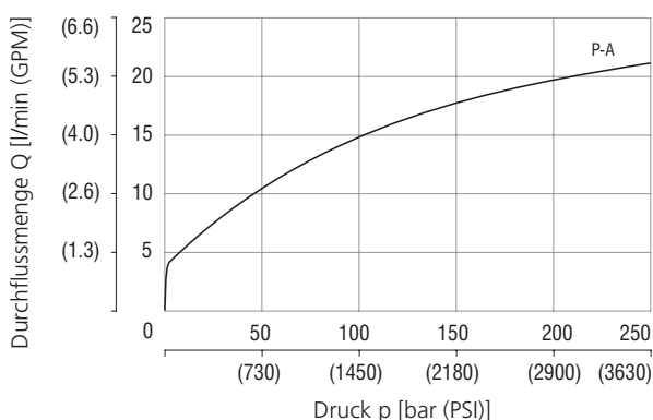
Leistungskennlinie SD2P-B4/H3Y13-5
