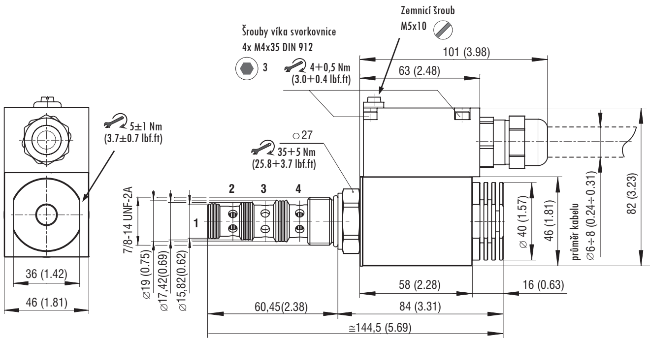
Rozměrový náčrt ventilu SD2PX-B4, rozměry v mm (in)
