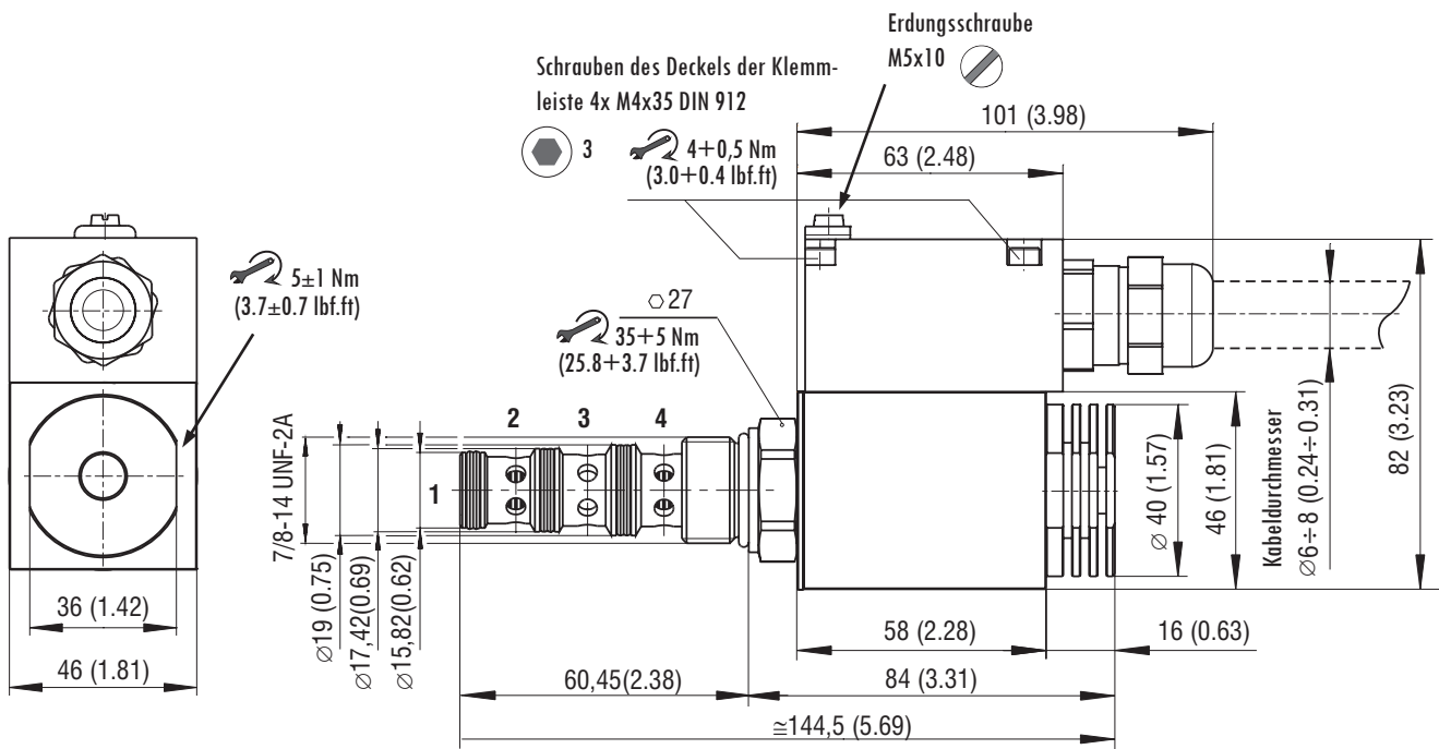
Maßskizze des Ventils SD2PX-B4, Abmessungen in mm (in)
