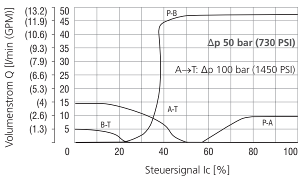
Leistungskennlinie SD2P-B4/H3Y13-5
