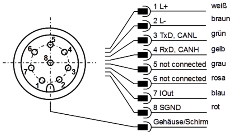
Abbildung 4.1: Pinbelegung bei Draufsicht auf den Sensordeckel
