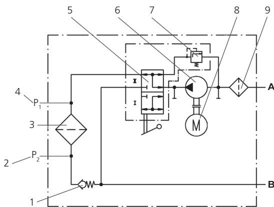
Abb. 12: Hydraulikschaltplan
