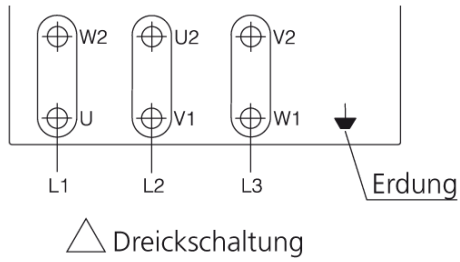
Abb. 13: Anschlussplan
