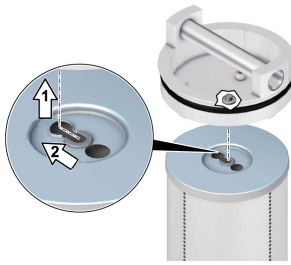
Abb. 6: Filterelement einhängen
