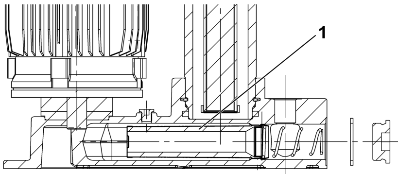
Abb. 10: Einbau des Saugfilterelements
