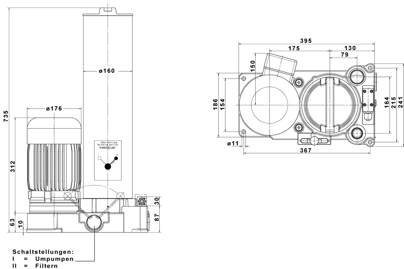
Abb. 11: Geräteabmessungen
