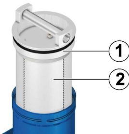
Abb. 7: Filterelement einbauen
