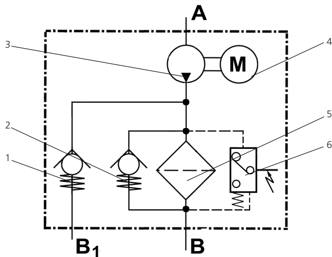
Abb. 10: Hydraulikschaltplan
