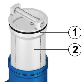
Abb. 4: Filterelement ausbauen
