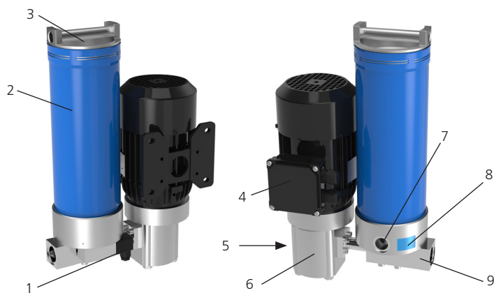
Abb. 1: Komponentenübersicht
