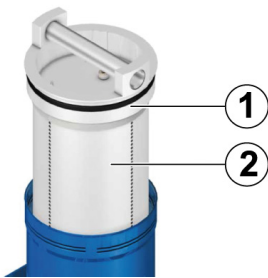
Abb. 7: Filterelement einbauen
