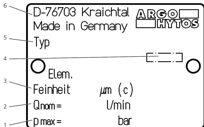
Abb. 2: Typenschild
