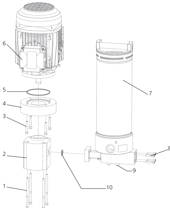
Abb. 8: Wechsel des Motors und der Pumpe
