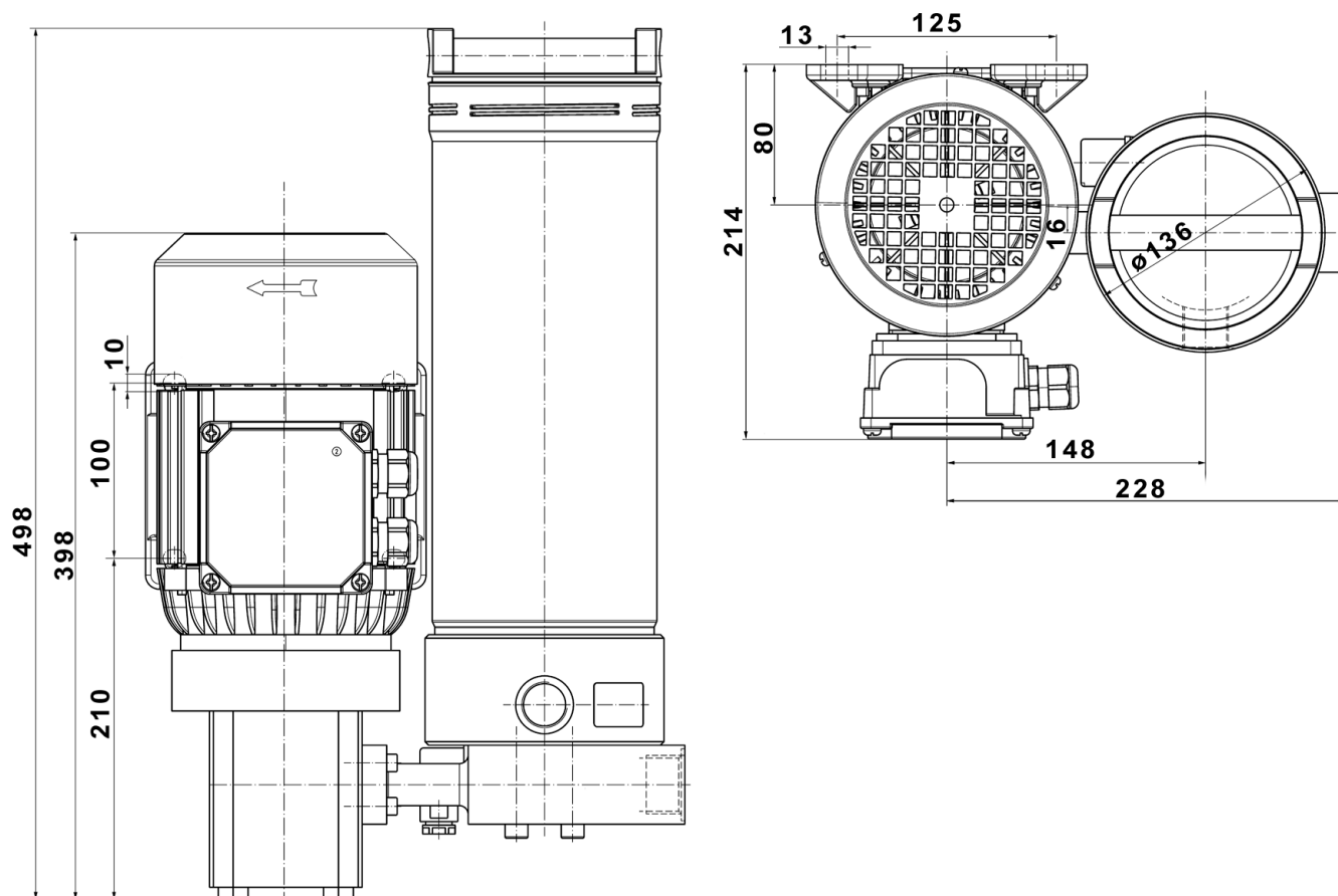
Abb. 9: Geräteabmessungen
