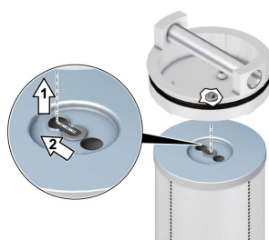
Abb. 6: Filterelement einhängen
