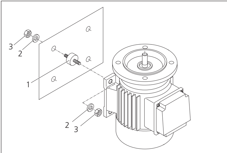
Abb. 3: Montagesatz
