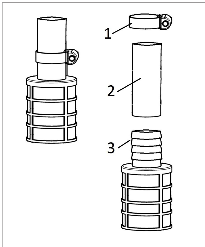
Abb. 8: Ansaugsieb FA 016.0303
