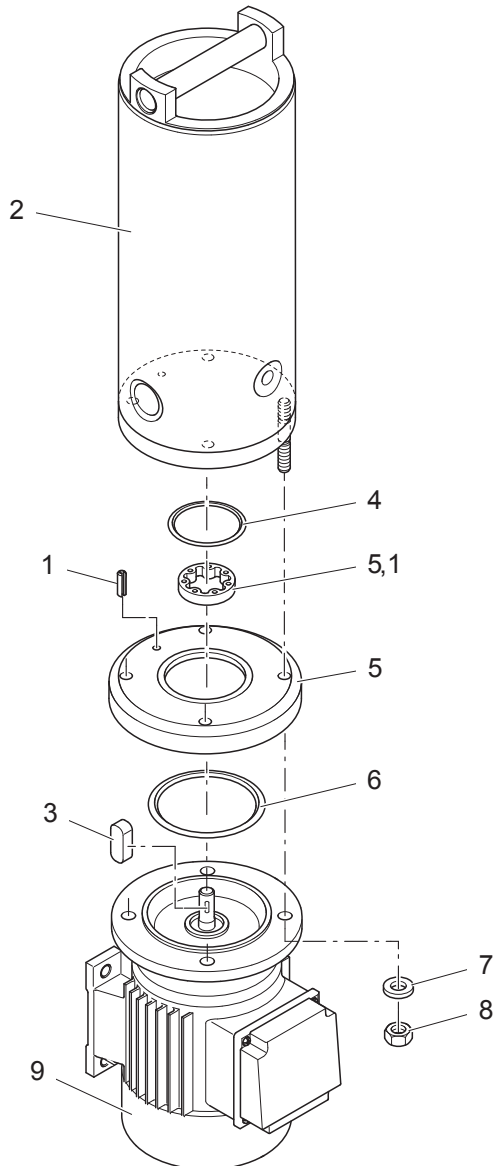
Abb. 5: Explosionsdarstellung der Nebenstromfiltereinheit
