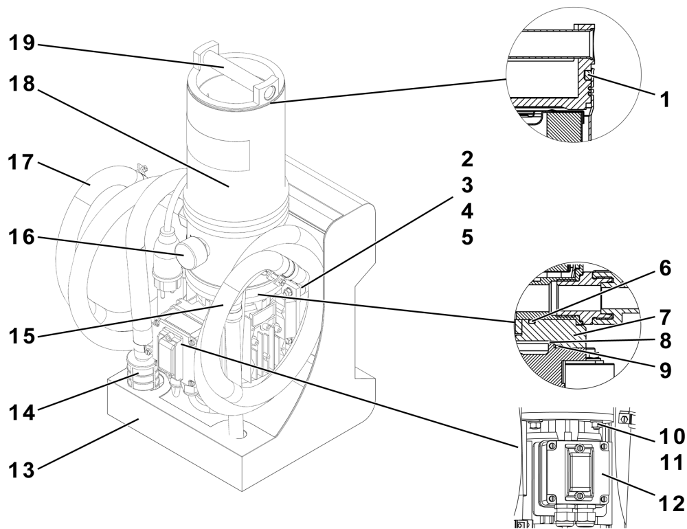
Abb. 13: Ersatzteilzeichnung
