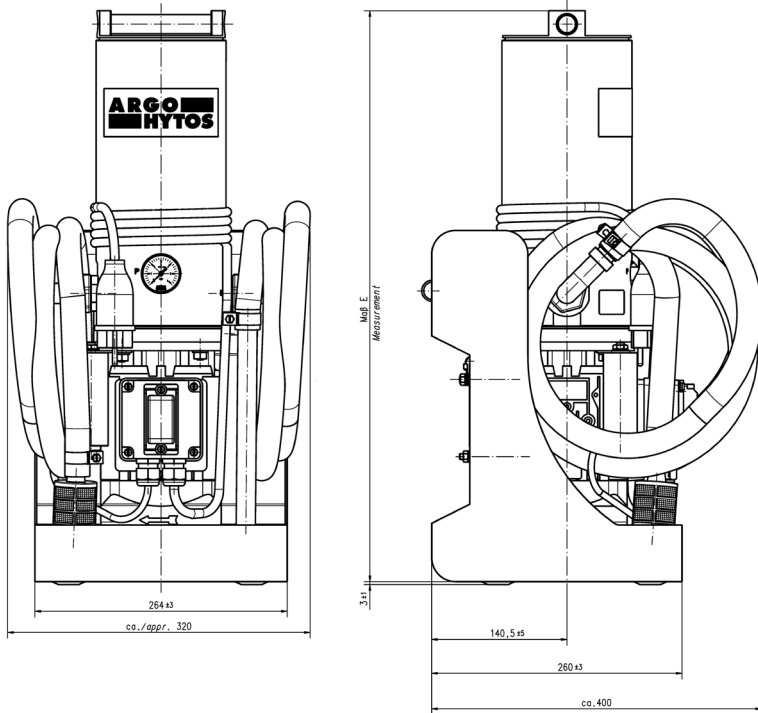
Abb. 11: Geräteabmessungen
