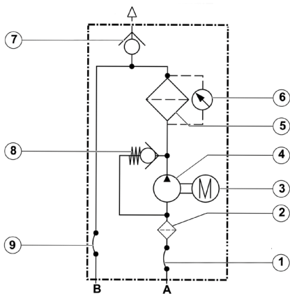
Abb. 12: Hydraulikschaltplan
