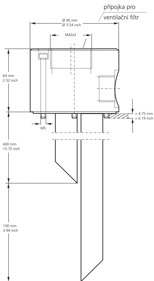
Montážní sada připevňená k nádrži
