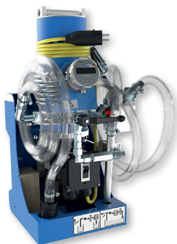
Agregát na údržbu oleje FAPC 016
