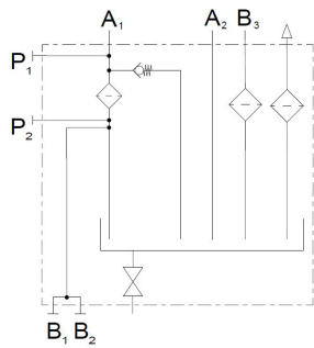
Rücklauffilter
