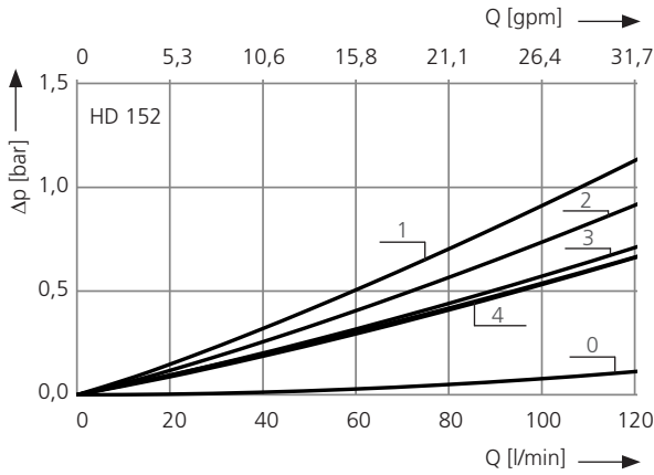
D1 Druckverlust in Abhängigkeit vom Volumenstrom bei v = 35 \text{ mm}^2/\text{s} / 162 SUS (0 = Gehäuse leer)
